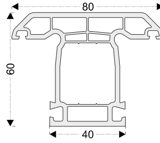
PRO03 Travesaño fijo
