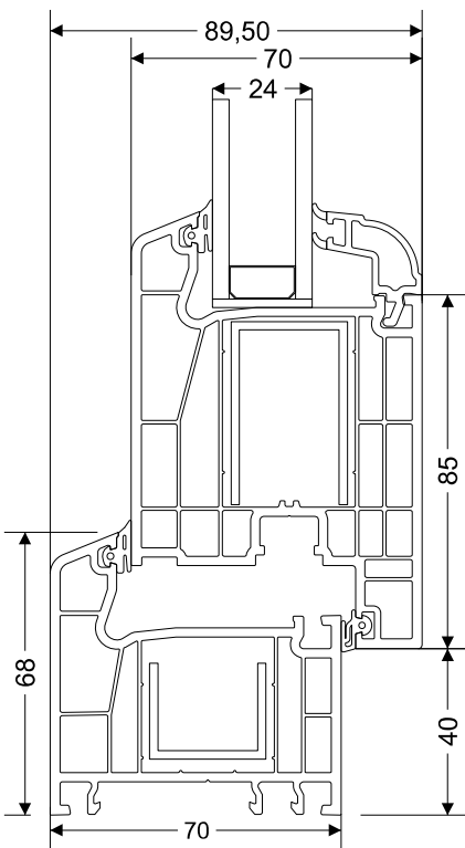
Marco - Hoja puerta apertura interna Conexión
