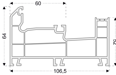
PRO23 Marco paño fijo
