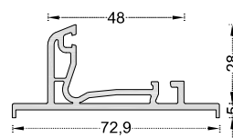
PRO201KA Adaptador fijo marco
