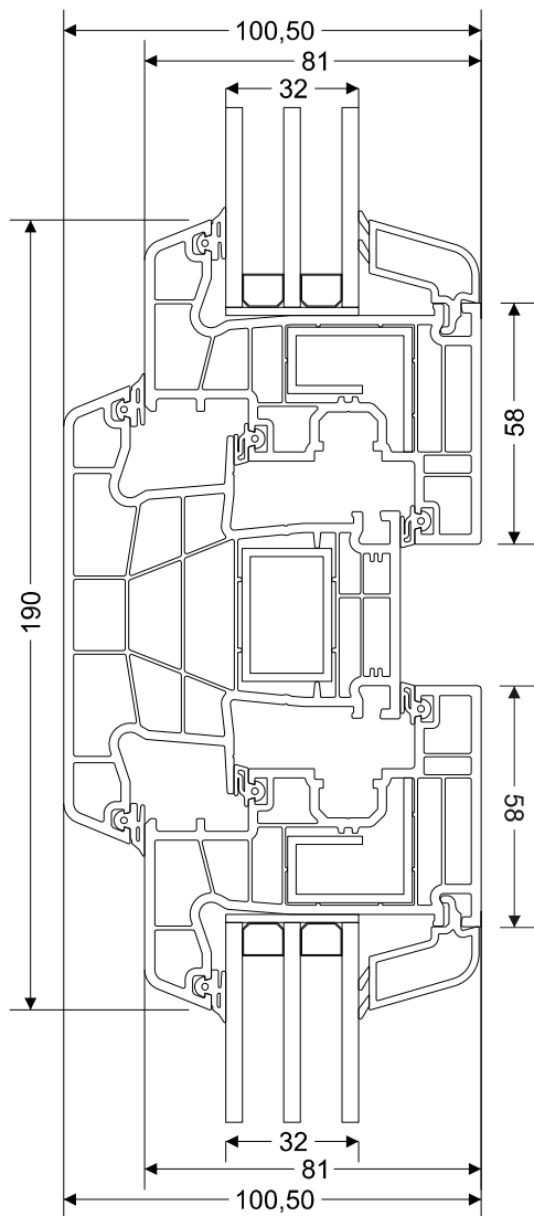
Hoja - Travesaño - Hoja
