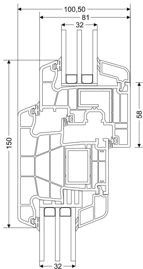
Travesaño - Hoja - Fijo
