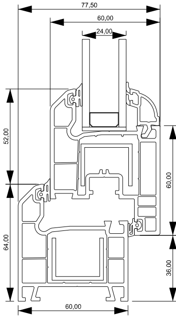
Marco - Hoja Conexión
