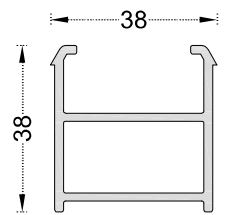
PRO1007 Perfil montaje marco
