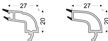
PRO701 Junquillo doble 20-22 mm
