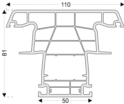
PRO8621 Travesaño fijo
