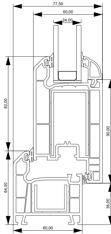
Marco - Hoja puerta apertura interior Conexión
