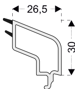
PRO8643 Junquillo triple 32 mm para hojas PRO8601, PRO8621
