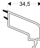
PRO8644 Junquillo doble 24 mm para hojas PRO8601, PRO8621
