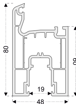
PRO211 Hoja puerta corrediza
