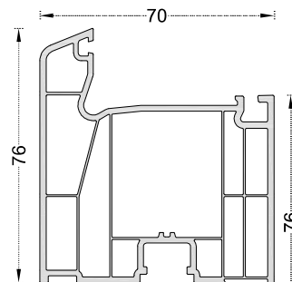
PRO718 Hoja puerta apertura interna
