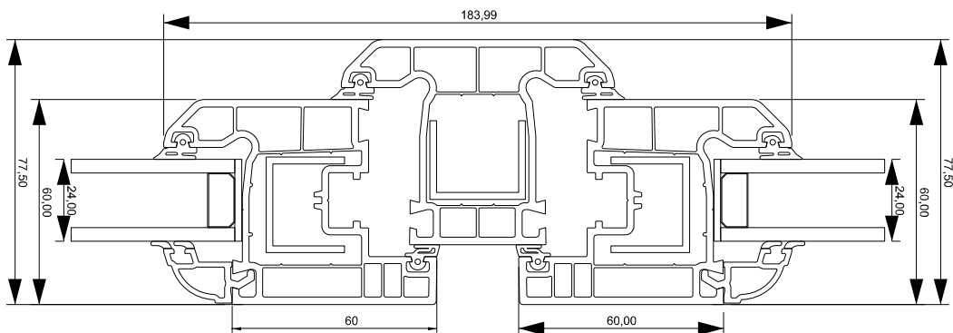
Hoja - Travesaño - Hoja Conexión
