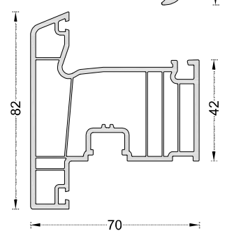
PRO722 Hoja apertura externa
