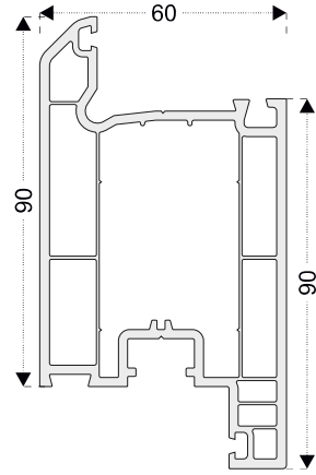
PRO04 Hoja puerta apertura interior
