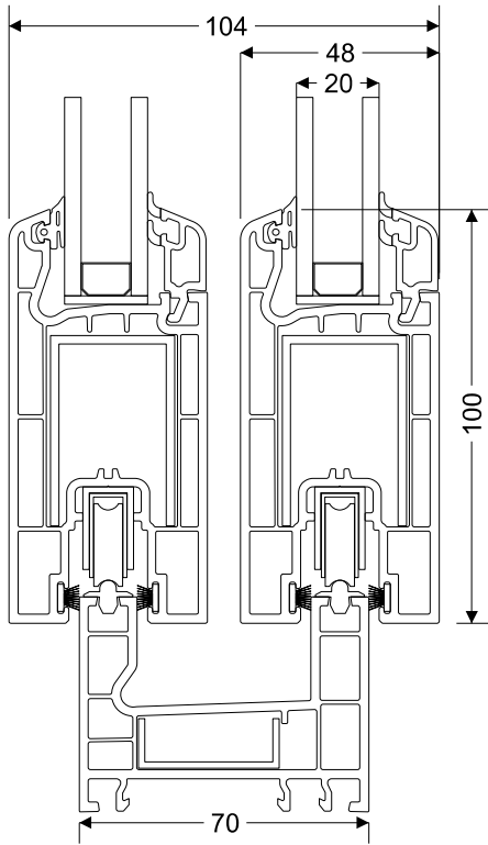
Marco 2 guías - Hoja corrediza
