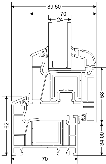
Marco 42 mm - Hoja Conexión
