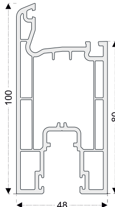
PRO213 Hoja puerta corrediza
