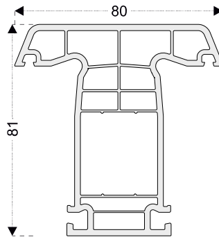
PRO8623 Travesaño fijo
