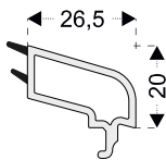
PRO8641 Junquillo triple 32 mm para hojas PRO8611, PRO8631
