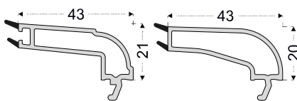
PRO700 Junquillo simple 4-6 mm
