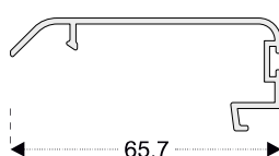
PRO43 Perfil de cierre marco 3 guías (alum.)
