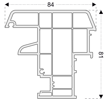
PRO8622 Travesaño móvil
