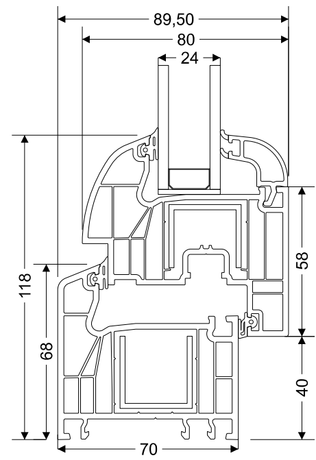
PRO7006 Marco (6 cámaras) Hoja semienrasada Conexión
