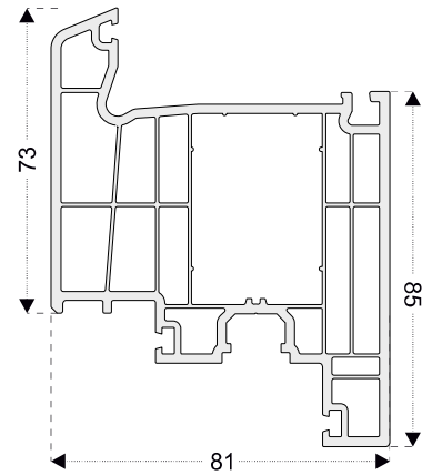
PRO8631 Hoja puerta apertura interna
