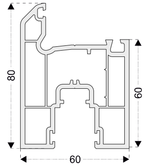
PRO21 Hoja corrediza
