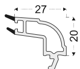
PRO205 Riel mosquitero (alum.)
