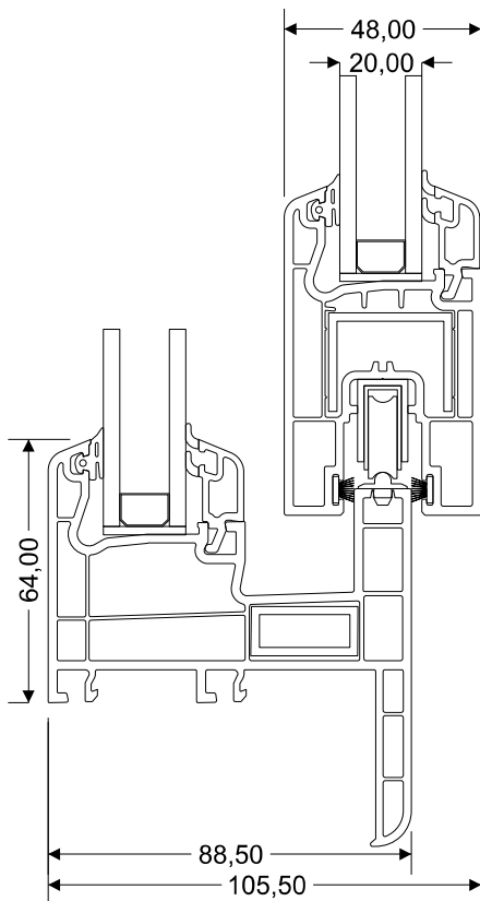
Marco paño fijo - Hoja corrediza
