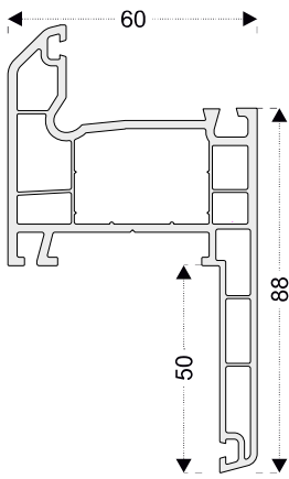
PRO82 Marco con solape
