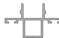
PRO411 Perfil de bloqueo hoja corrediza (alum.)
