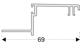
PRO28 Perfil de cierre marco 2 guías (alum.)
