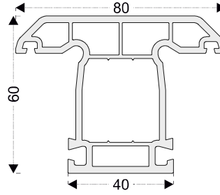
PRO53 Travesaño fijo
