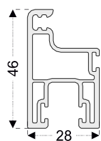
PRO234 Hoja corrediza mosquitero
