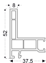
PRO205 Riel mosquitero (alum.)
