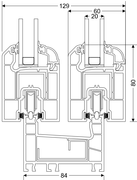
Marco - Hoja corrediza 80 mm
