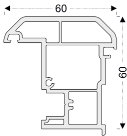
PRO12 Travesaño móvil
