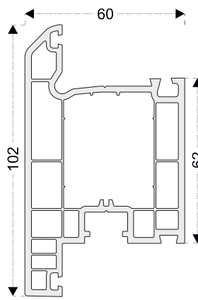
PRO10 Hoja puerta apertura exterior
