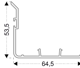
PRO25 **para PRO24 Adaptador hoja corrediza
