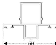
PRO41 Perfil de bloqueo hoja corrediza (alum.)
