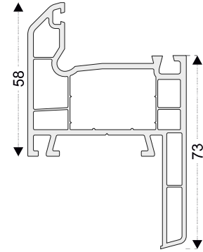
PRO81 Marco con solape
