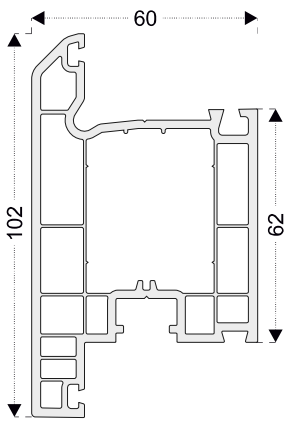
PRO10 Hoja puerta apertura exterior
