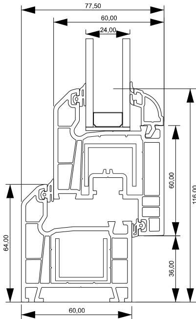
Marco - Hoja Conexión
