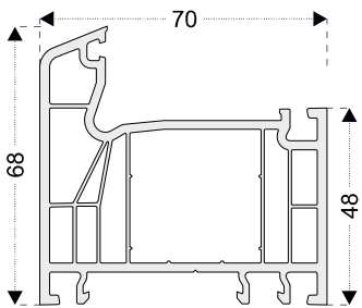
PRO720 Marco (6 cámaras)
