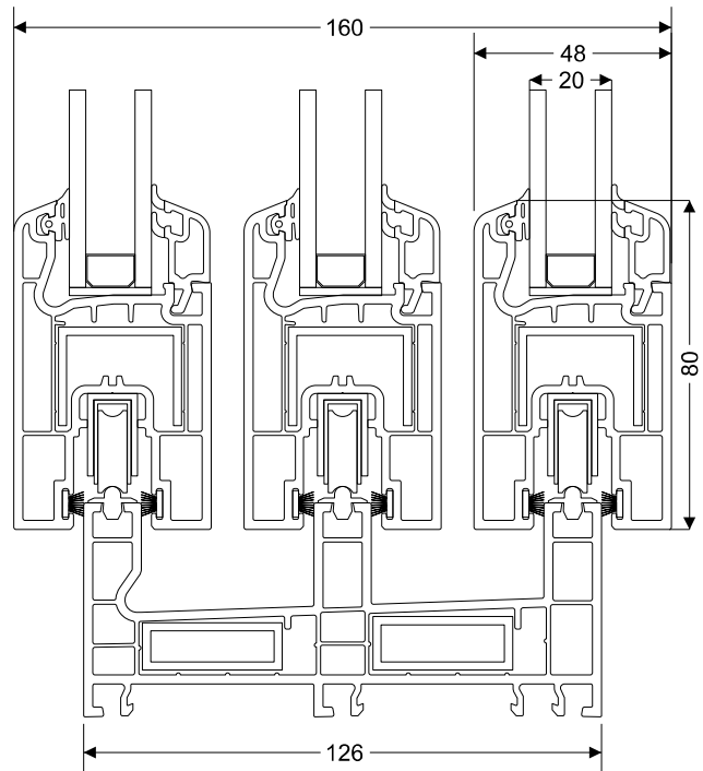
Marco 3 guías - Hoja corrediza
