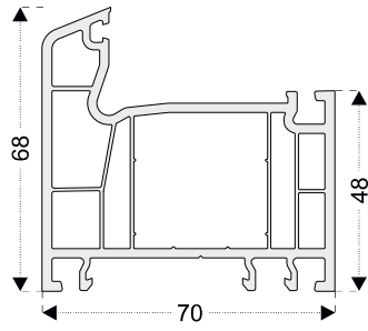
PRO710 Marco - 48 mm
