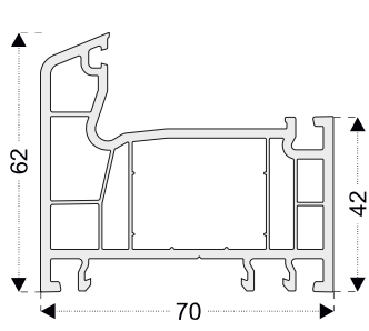
PRO711 Marco - 42 mm
