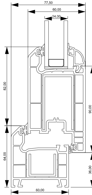
Marco - Hoja puerta interior Conexión
