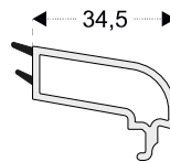
PRO8642 Junquillo triple 32 mm para hojas PRO8611, PRO8631
