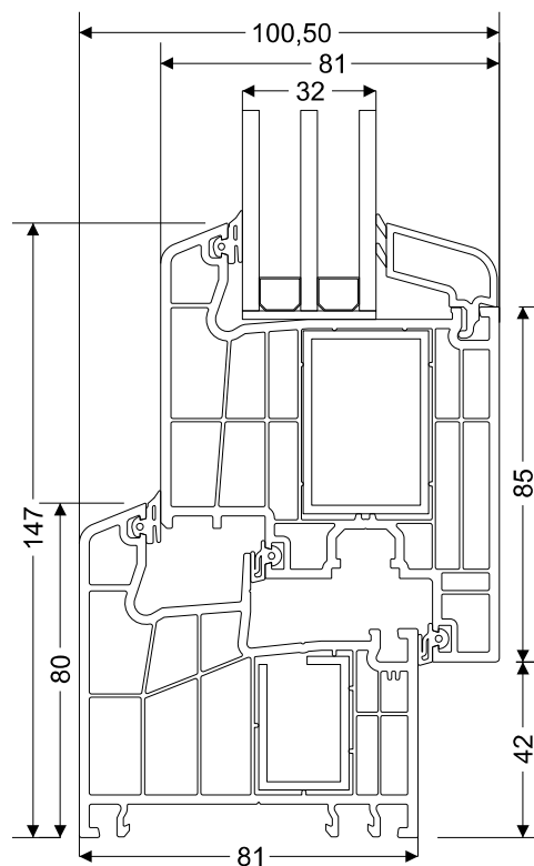
Marco - Hoja puerta apertura interna - Hoja Conexión
