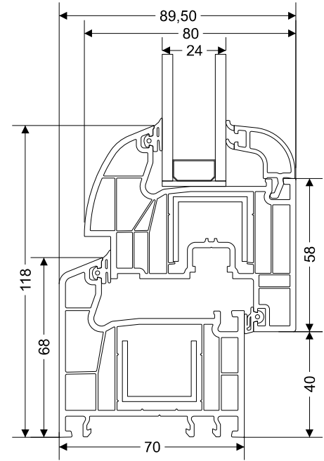
Marco - Hoja semienrasada Conexión
