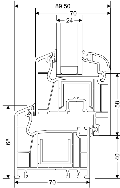
Marco 48 mm - Hoja Conexión
