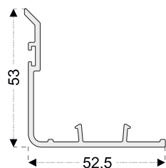
PRO214 ** para PRO213 Traslapo corredera
