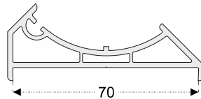
PRO331 Esquinero rótula 70 mm
