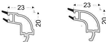
PRO702 Junquillo doble 24-26 mm
