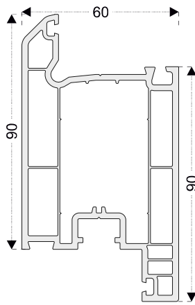
PRO04 Hoja puerta apertura interior
