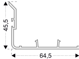
PRO22 **para PRO21 Adaptador hoja corrediza
