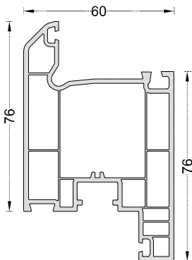
PRO523 Hoja puerta apertura interior
