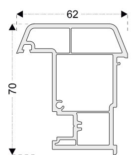
PRO717 Travesaño móvil
