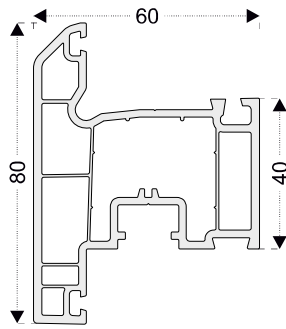
PRO521 Hoja ventana apertura exterior
