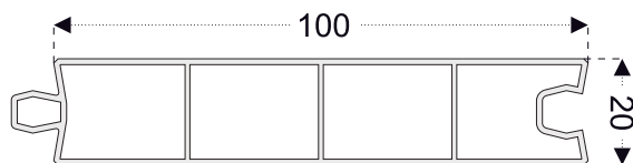
PRO30 Panel (Lambri) Profile
