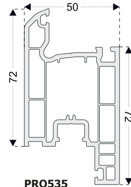
PRO535 Inward Door Profile
