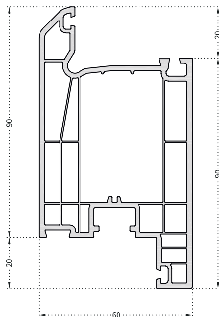
PRO17 6004 Door Sash
