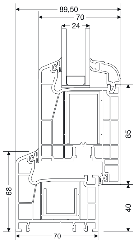
Frame - Inward Door Sash Connection Section
