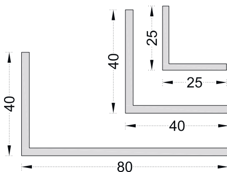
PRO1004 25x25 Köşebent Profili
