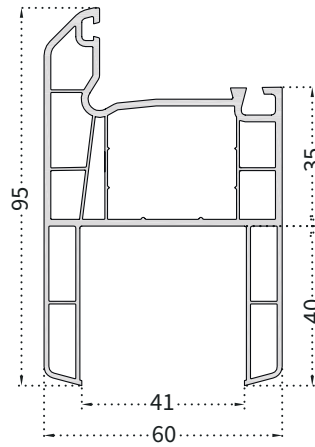
PRO15 6004 Konteyner Kasa
