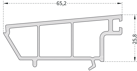
PRO1402 Sürme Kasa Kapama
