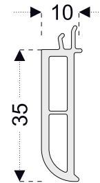
PRO39 Tırnaklı Pervaz (70mm Seri)
