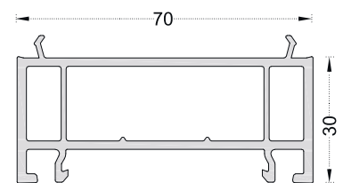
PRO1008 30mm Yükseltme (70 mm Seri)
