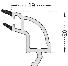
PRO05 4mm Cam Çıtası
