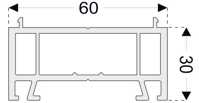
PRO14 30 mm Yükseltme (60 mm Seri)
