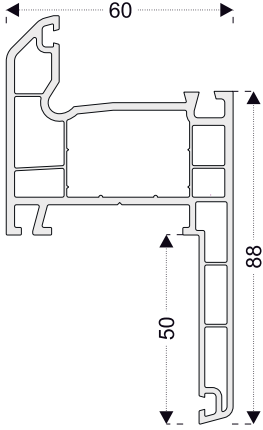
PRO82 Pervazlı Kasa
