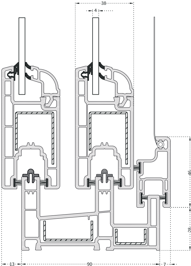
Sürme Sineklikli Kasa (Sineklik İçte) - Sürme Kanat Kesit Detayı
