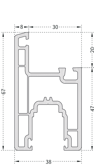
PRO604 60mm Sürme Kanat (67 mm)
