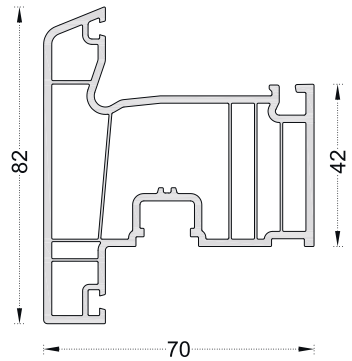
PRO722 T Kanat
