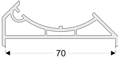
PRO331 Köşe Dönüş Adaptörü - 70mm
