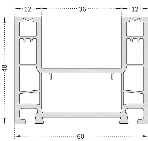
PRO600 60mm Çift Ray Sürme Kasa
