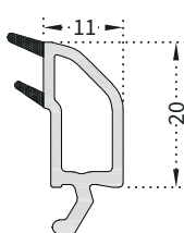
PRO07 12mm Cam Çıtası
