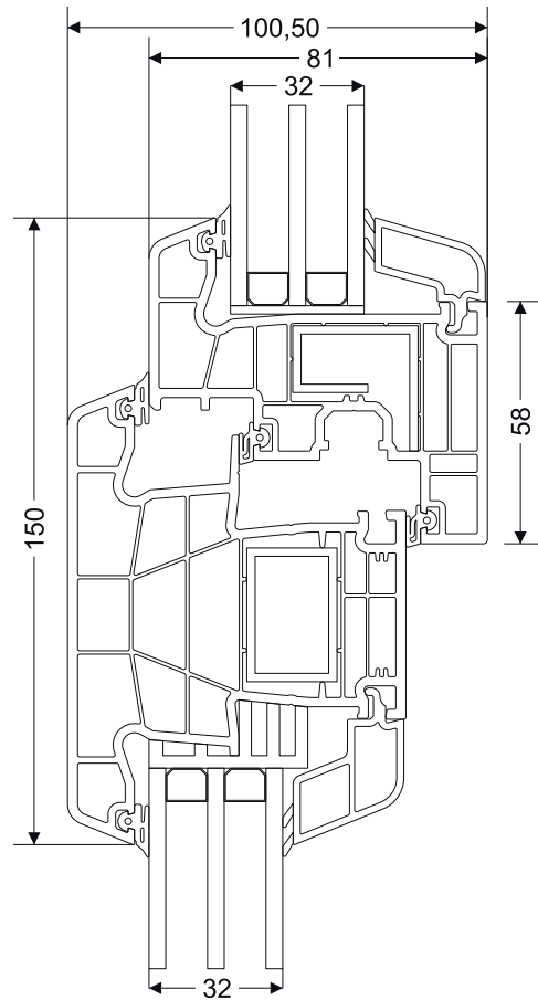
Kanat - Orta Kayıt - Sabit
