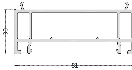
PRO8639 30 mm Yükseltme (81 mm Seri)
