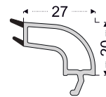
PRO701 20-22 mm Cam Çıtası
