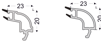
PRO702 24-26 mm Cam Çıtası
