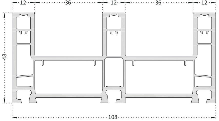
PRO601 60mm Üçlü Sürme Kasa
