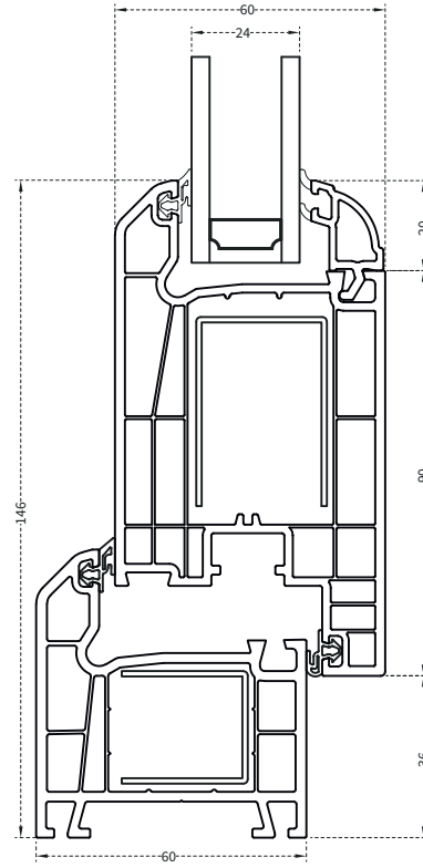
Kasa - İç Açılan Kapı Kanat Kesit Detayı
