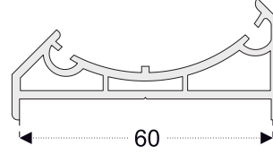
PRO33 Köşe Dönüş Adaptörü - 60mm
