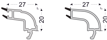
PRO701 20-22 mm Çift Cam Çita
