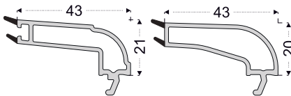
PRO700 4-6 mm Cam Çıtası
