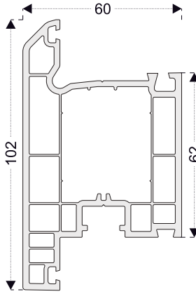
PRO10 T Kapı Kanat
