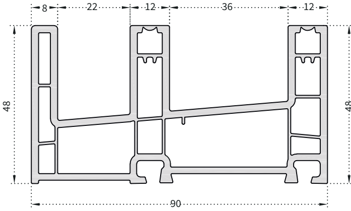
PRO602 60mm Sürme Sineklikli Kasa (Sineklik Dışta)
